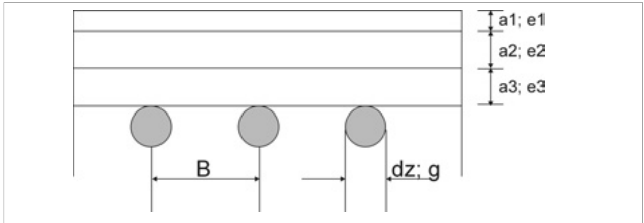
Рис. 2. Величины, характеризующие конструкцию нагревателя.
